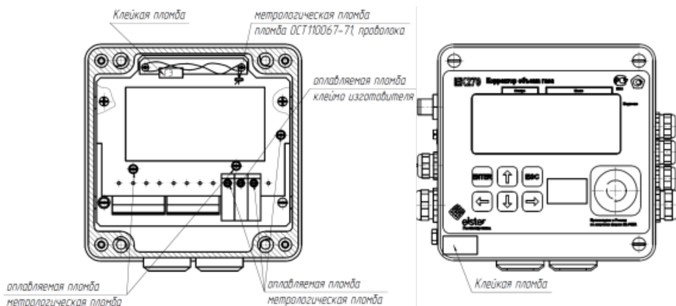
Рис. 3 Расположение пломб
